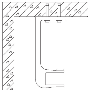
Eksempel på beslag montert i tak
