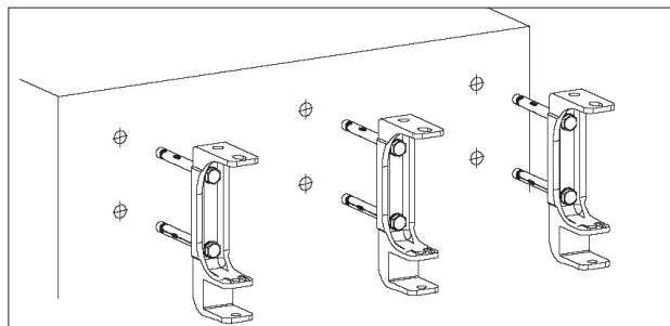
Eksempel på beslag montering på murvegg
